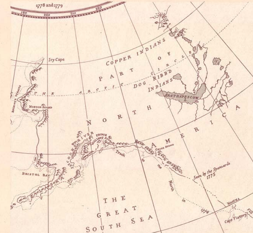
Cook 1784
