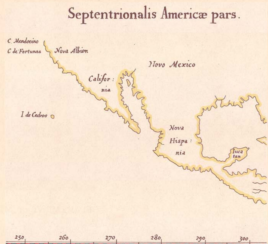
De Laet 1630
