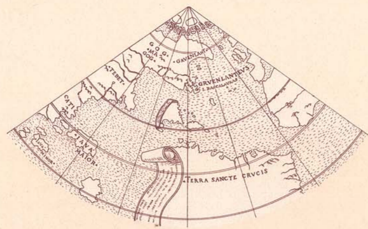
Ruysch 1508
