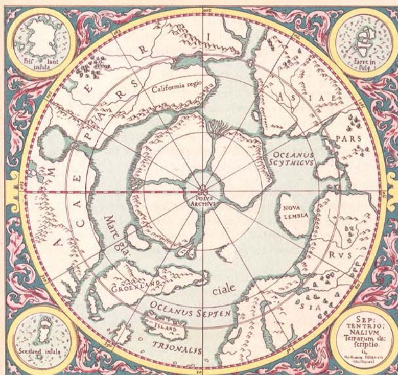
Mercator 1595
