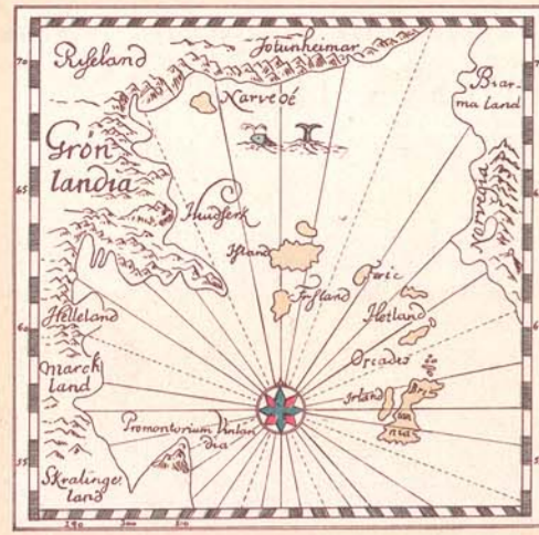
Stephanus 1590
