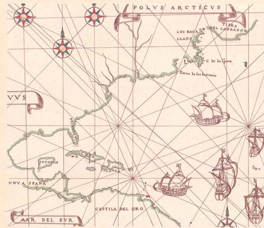
Ribero 1529
