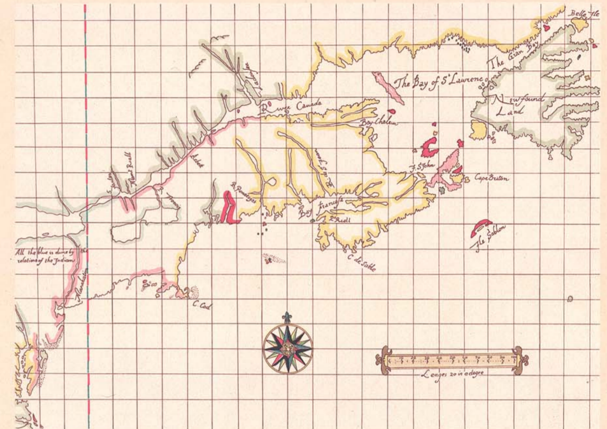
Velasco 1610
