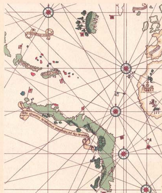
Cancero 1502-04
