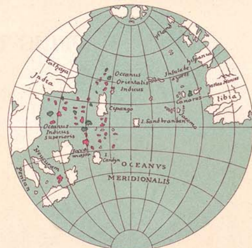
Behaim 1492
