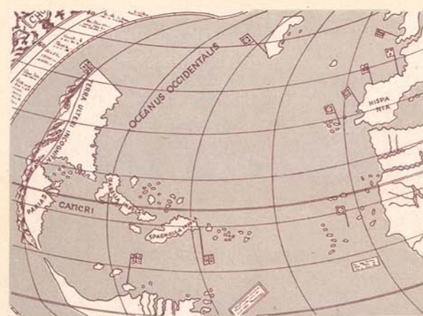
Waldseemüller 1507
