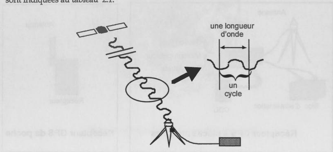
Figure 2.4 Onde porteuse
