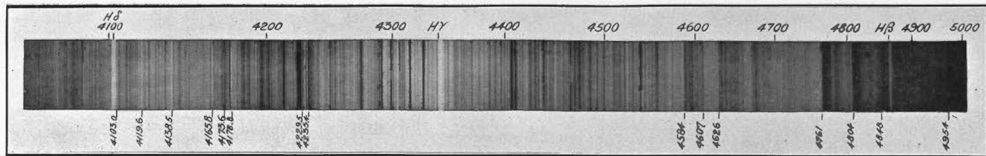
Spectrum of O Ceti (Mira).
