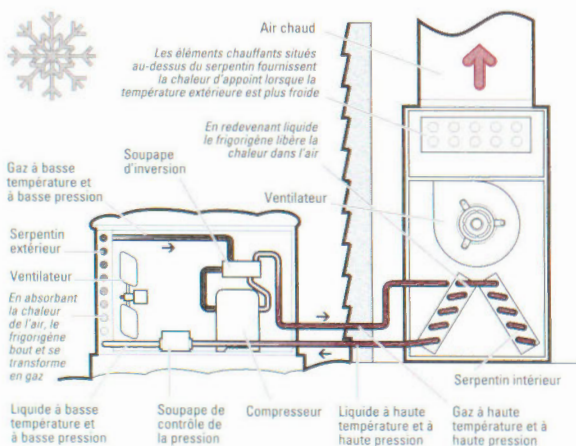
Figure 13 : Thermopompe à air en mode chauffage
