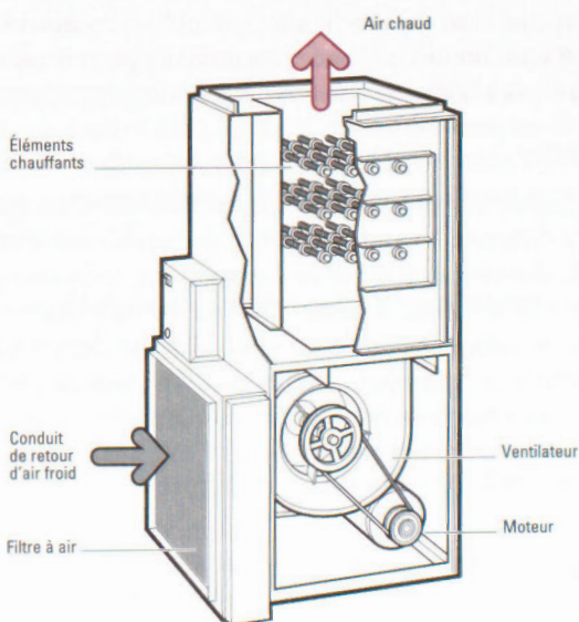
Figure 2 : Générateur d'un système électrique à air pulsé
