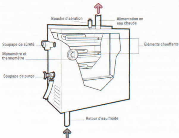
Figure 5 : Chaudière d'un système hydronique
