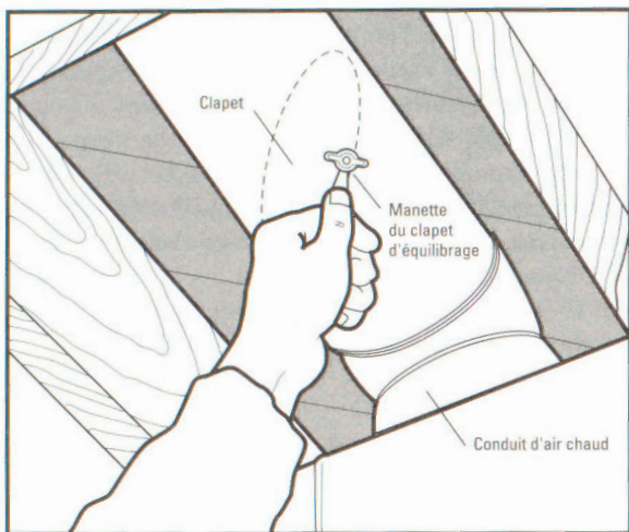
Figure 4 : Clapet d'équilibrage du conduit d'alimentation
