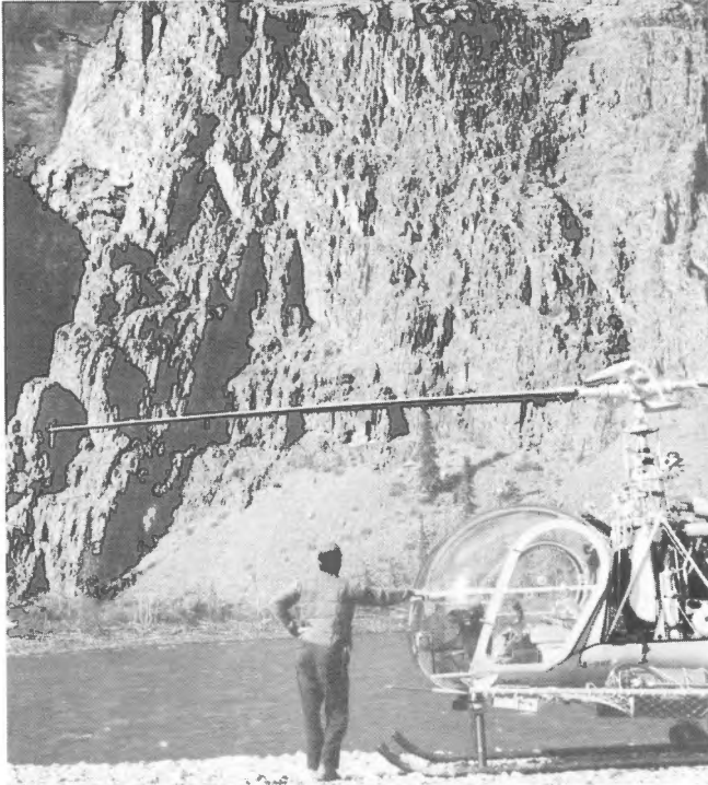
Un géologue observe sur une paroi rocheuse, les effets de l'érosion qui a causé un éboulis à la base.
