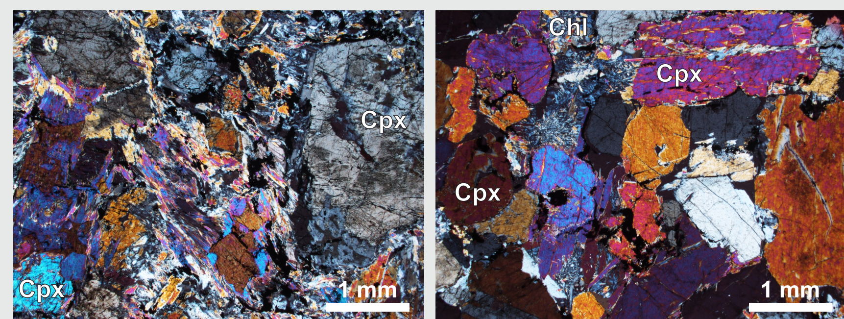
Photo 1. Clinopyroxénite avec clinopyroxènes (Cpx) xénomorphes dans une matrice d'amphibole et clinopyroxènes (Cpx) avec chlorite chlorite (lumière polarisée analysée = LPA)
