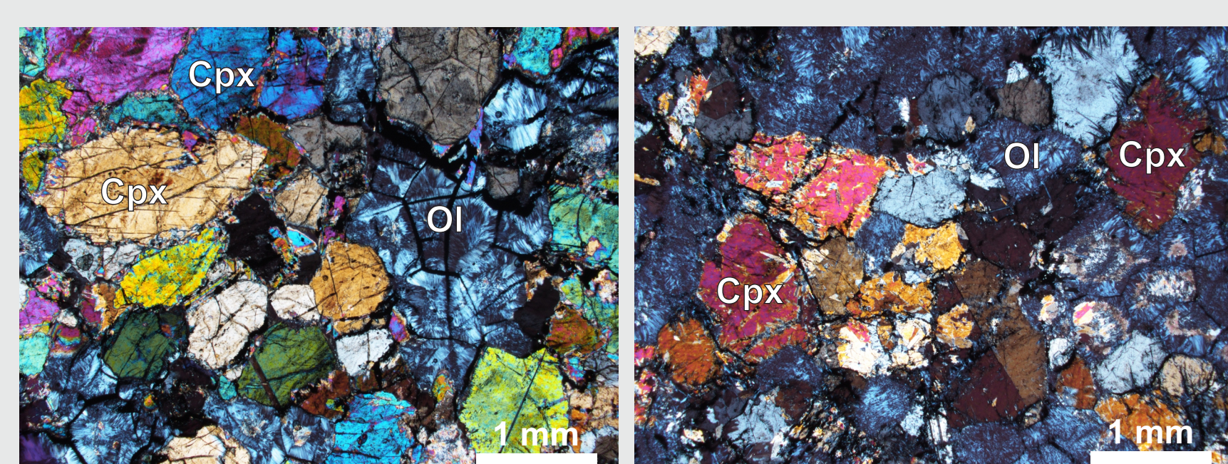
Photo 2. Clinopyroxénite à olivine. Orthocumulat à olivine (Ol) serpentinisée avec serpentinisée avec clinopyroxènes (Cpx) interstitiels (LPA)
