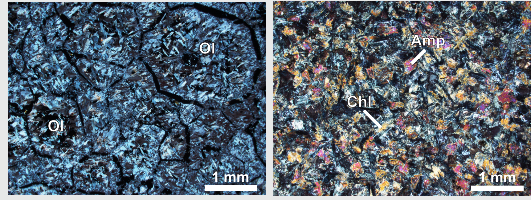
Photo 3. Wehrilite. Orthocumulat à olivine (Ol) serpentinisée avec serpentinisée avec clinopyroxènes (Cpx) interstitiels (LPA)
