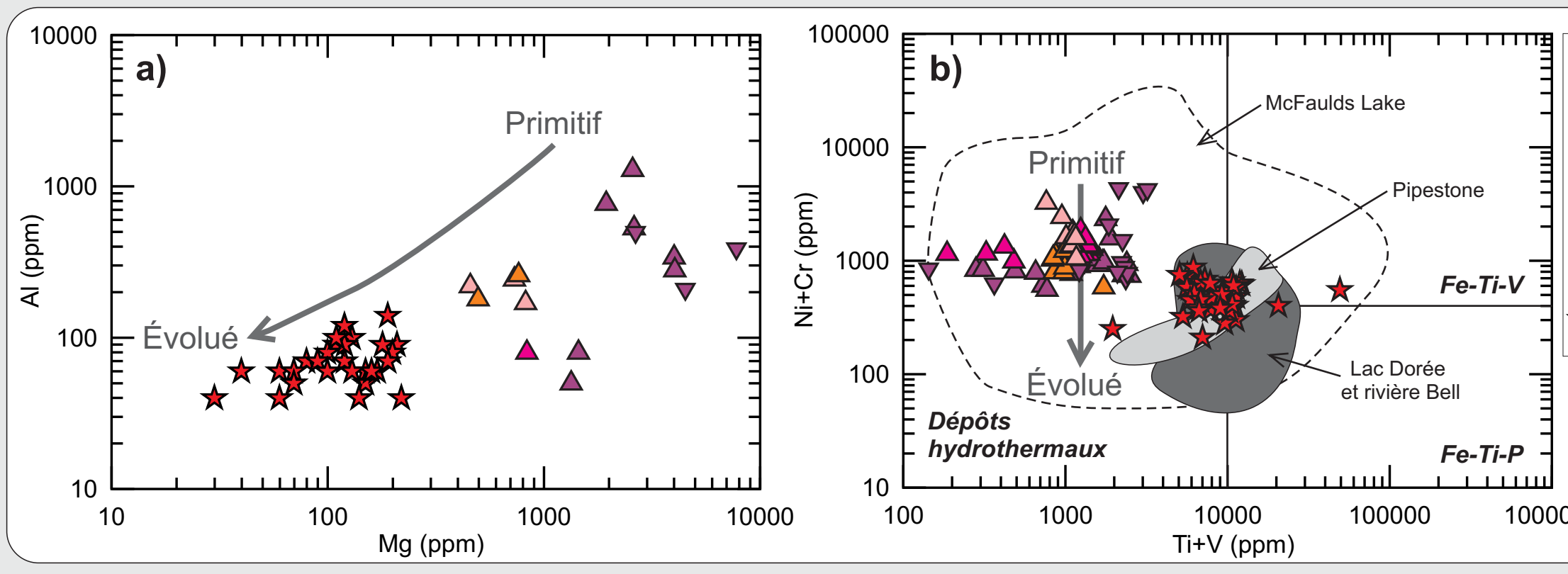
Fig. 6. Compositions des magnétites (analyses individuelles) en fonction des principales subdivisions géographiques de la Pyroxénite de baie Chapus (voir Fig. 2b). a) Al vs Mg et b) Ni+Cr vs Ti+V (diagramme d'après Méric, 2011). Champs des magnétites dans les intrusions de McFaulds Lake (ON) et des complexes du lac Doré et de la rivière Bell (QC) définis d'après des données non publiées (Kuznick, 2014; Sappin, 2014). Champ des magnétites dans Complexe anorthositique de Pipestone Lake (MA) défini d'après Jobin-Bevans (1997).
