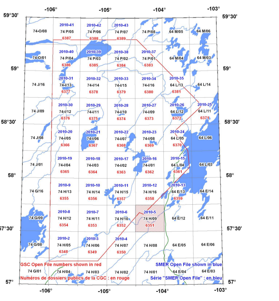
AIRBORNE GEOPHYSICAL SURVEY OF THE EASTERN ATHABASCA BASIN, SASKATCHEWAN LEVÉ GÉOPHYSIQUE AÉROPORTÉ DE LA PARTIE EST DU BASSIN ATHABASCA, SASKATCHEWAN
