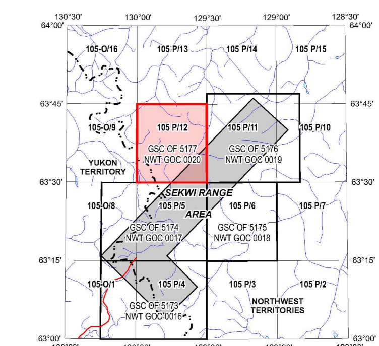
NATIONAL TOPOGRAPHICAL SYSTEM REFERENCE AND GEOGRAPHICAL MAP INDEX SYSTÈME NATIONAL DE RÉFÉRENCE CARTOGRAPHIQUE ET INDEX DES CARTES GÉOGRAPHIQUES
