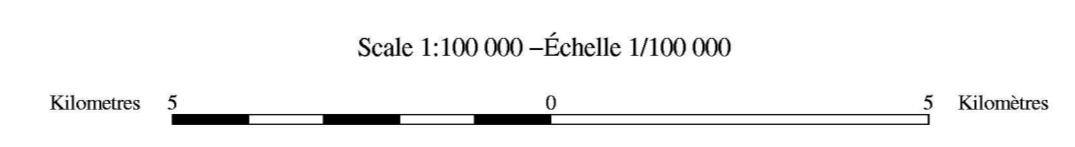
AEROMAGNETIC TOTAL FIELD MAP CARTE AÉROMAGNÉTIQUE DU CHAMP TOTAL 106 P/SW-SE NORTHWEST TERRITORIES TERRITOIRES DU NORD-OUEST
