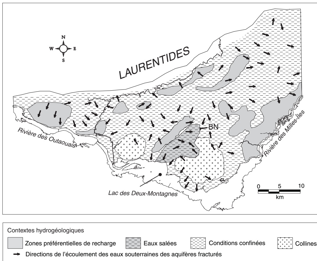
Figure 4. Contextes hydrogéologiques et directions d'écoulement des eaux souterraines. BN = Saint-Benoît.
