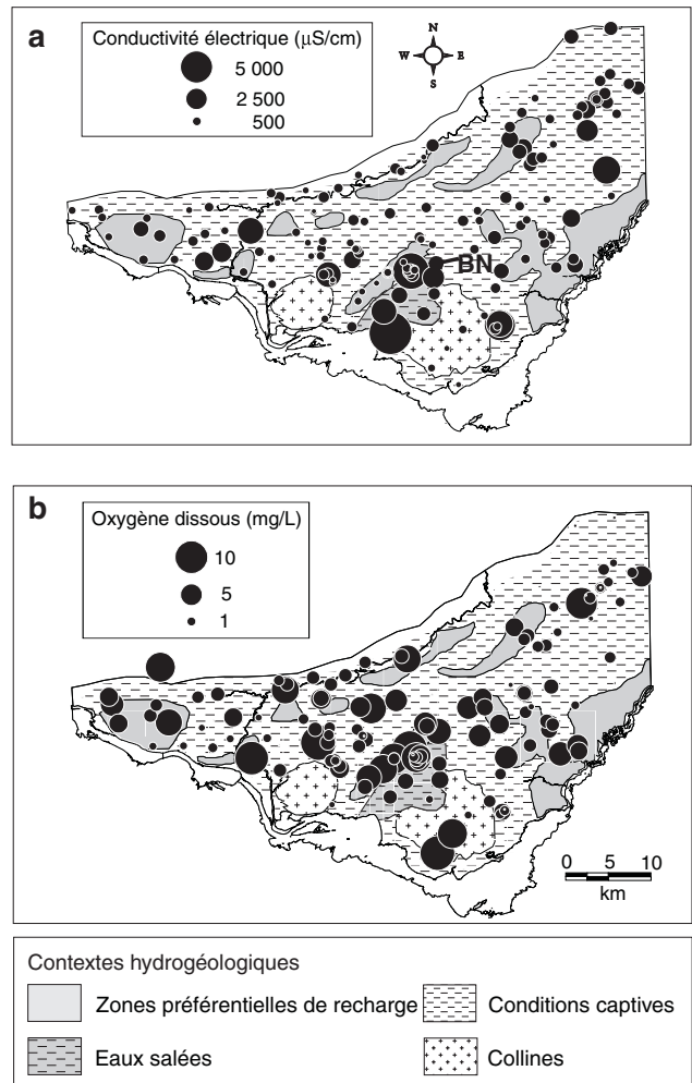
Figure 6. Distribution régionale des conditions géochimiques de l'eau souterraine; a) conductivité électrique à 25 °C; b) oxygène dissous (échantillons de 1999 et 2000). BN = Saint-Benoît.
