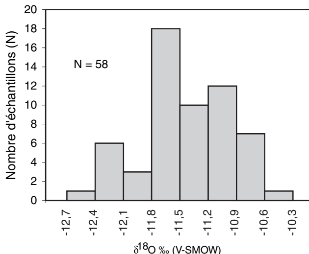
Figure 9. Distribution de fréquence de δ 18 O dans l'eau souterraine.
