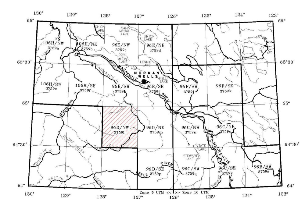
NATIONAL TOPOGRAPHIC SYSTEM REFERENCE AND GEOPHYSICAL INDEX FOR GEOLOGICAL SURVEY OF CANADA MAPS SYSTÈME NATIONAL DE RÉFÉRENCE CARTOGRAPHIQUE ET D'INDEX DES CARTES GÉOPHYSIQUES POUR LA COMMISSION GÉOLOGIQUE DU CANADA
