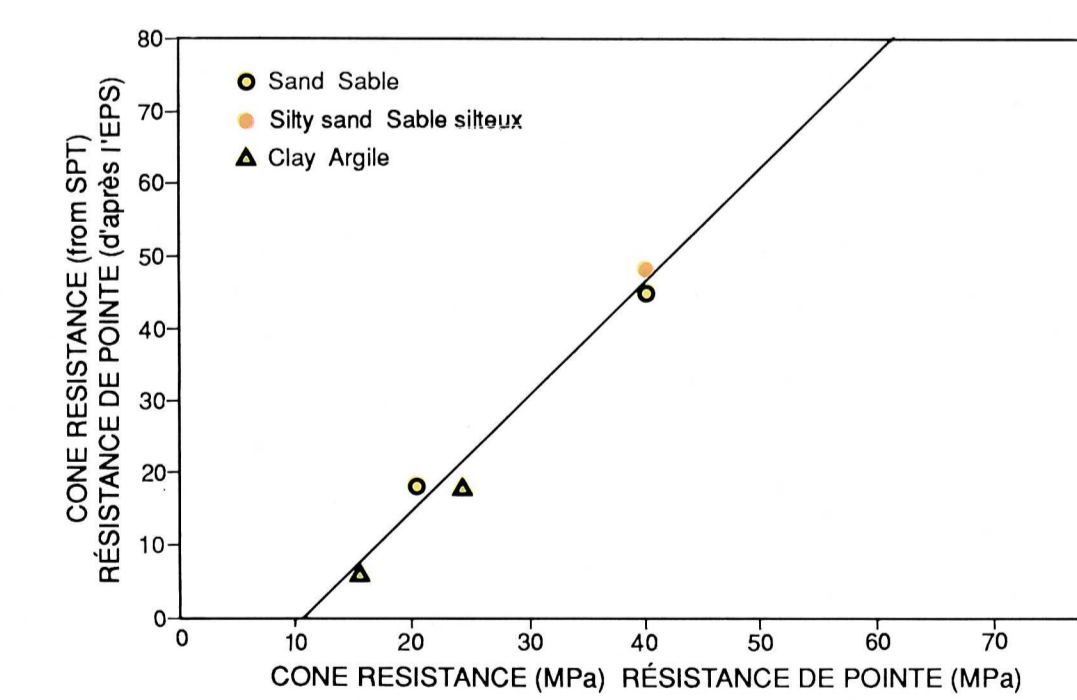
FIGURE 11. Comparison of Sabie Island Bank cone penetrometer resistance with equivalent resistance estimated from standard penetration tests from Georges Bank FIGURE 11. Comparaison entre la résistance de pointe relevée au banc de file de Sabie à l'aide d'un pénétromètre et la résistance équivalente estimée d'après des essais de pénétration standard dans le banc de Georges
