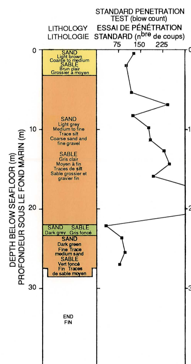
FIGURE 5. Propriétés physiques du sondage 1, site 2
