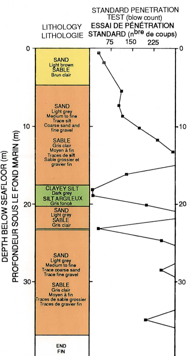
FIGURE 4. Propriétés physiques du sondage 3, site 1
