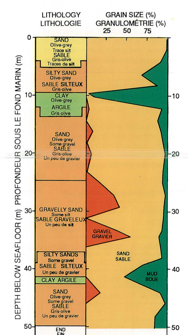
FIGURE 10. Propriétés physiques du sondage, site de Louisbourg, Le Banquerneau
