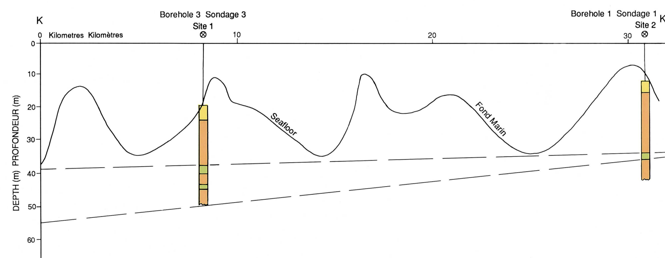
FIGURE 6. Coupe transversale K-K' recoupant le sondage 3 (site 1) et le sondage 1 (site 2)
