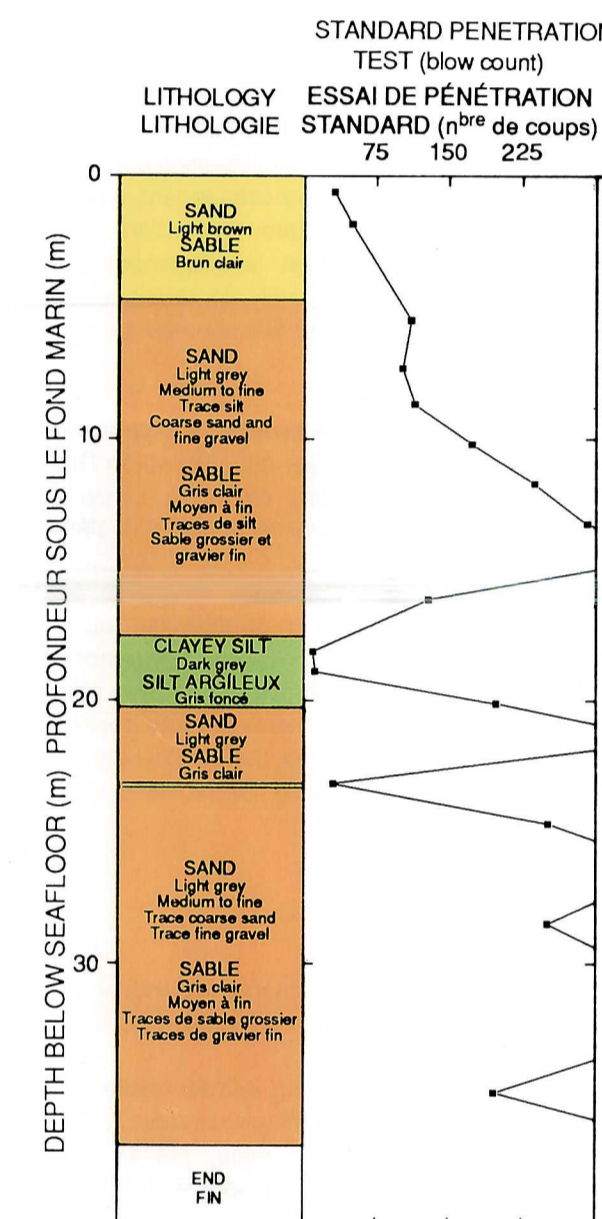
FIGURE 8. Propriétés physiques du sondage 3, site 1, banc de Georges
