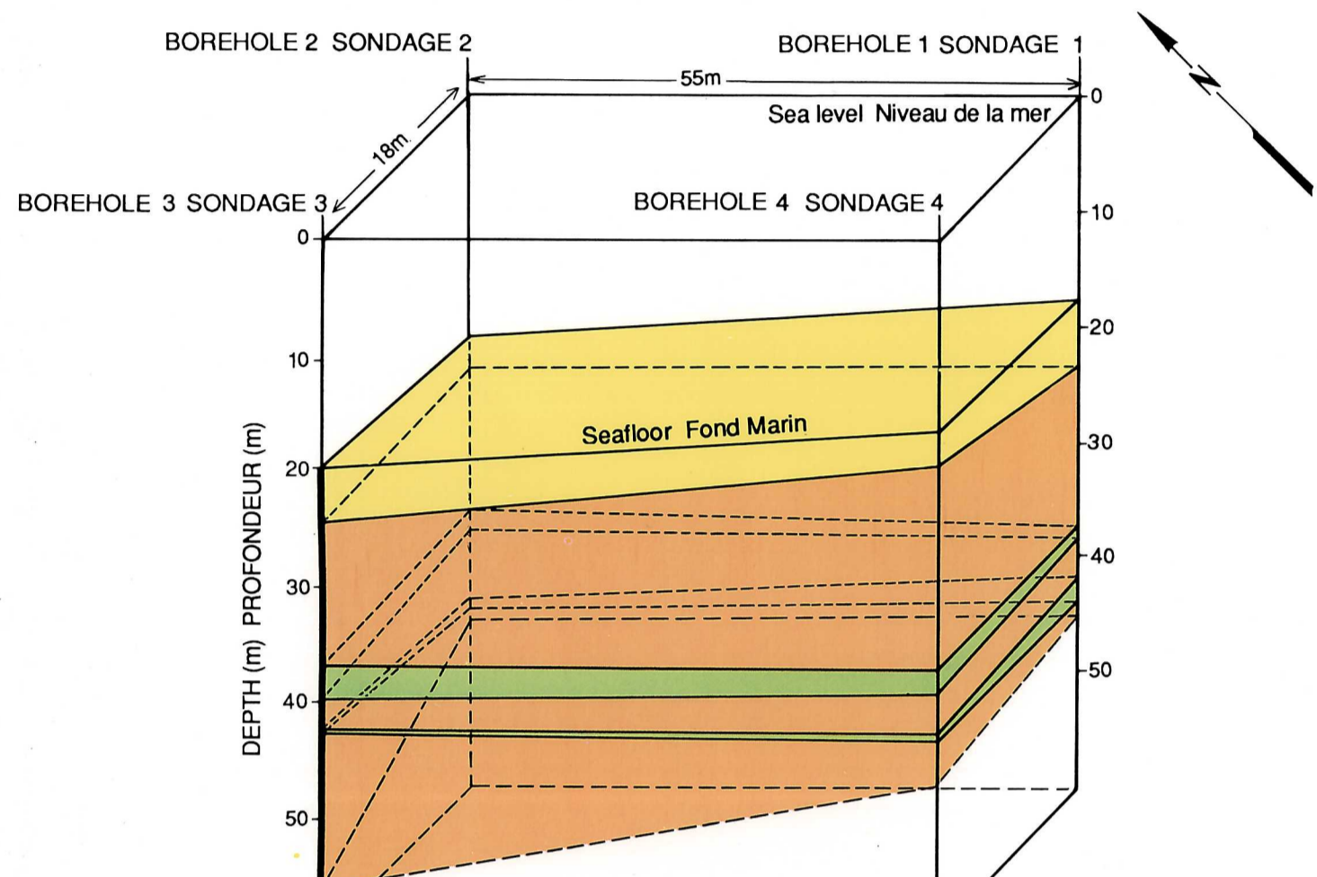
FIGURE 2. Coupe tridimensionnelle du site 1 délimitée par les sondages 1, 2, 3 et 4
