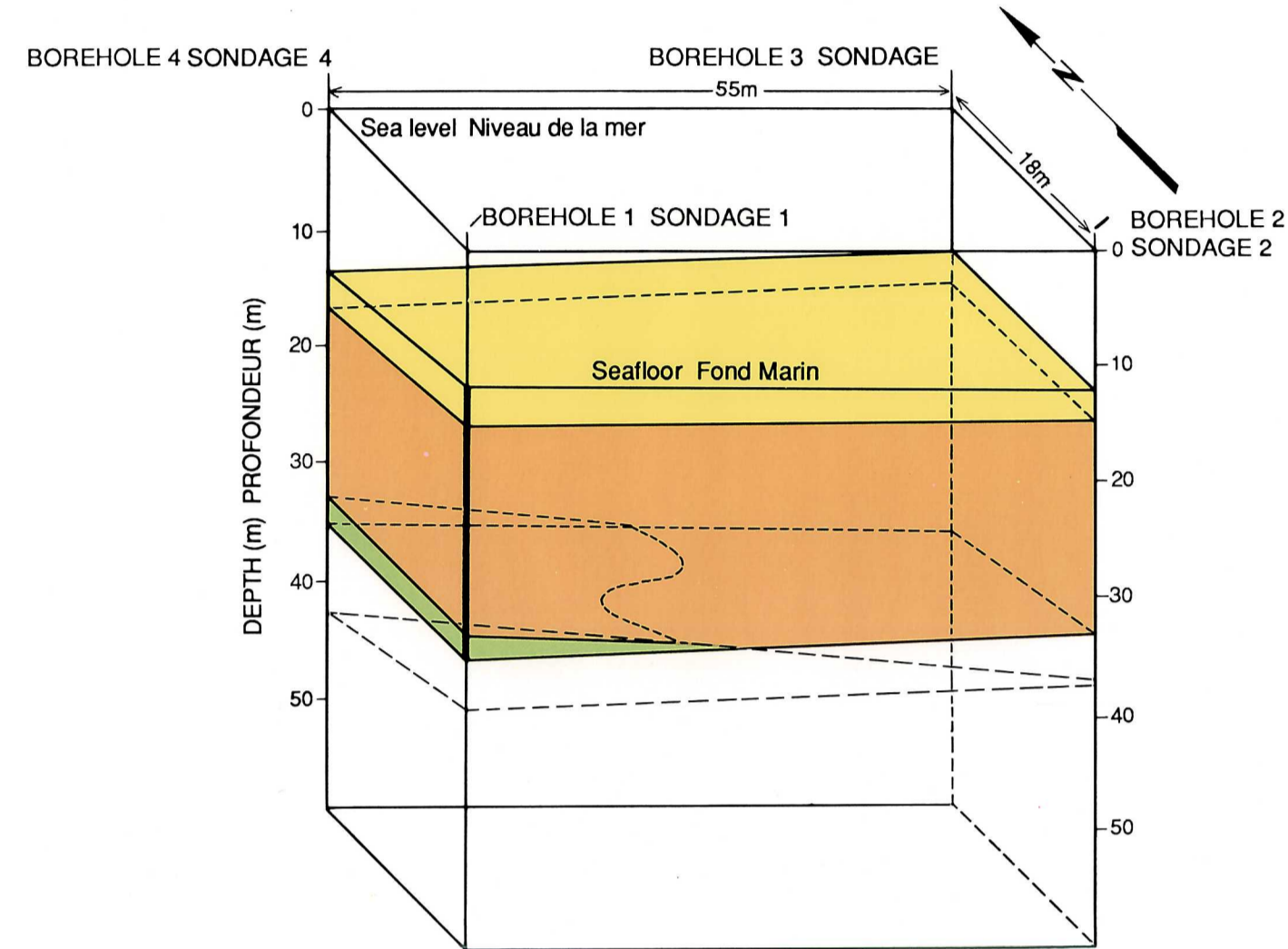
FIGURE 3. Coupe tridimensionnelle du site 2 délimitée par les sondages 1, 2, 3 et 4
