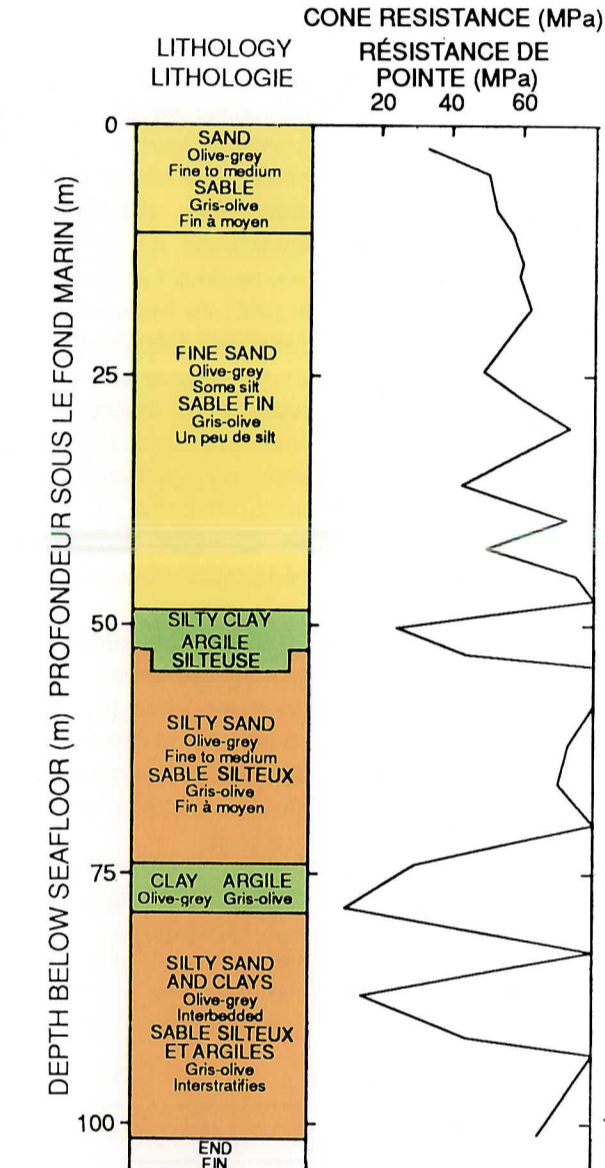
FIGURE 9. Propriétés physiques du sondage C-2, Venture central, banc de file de Sabie
