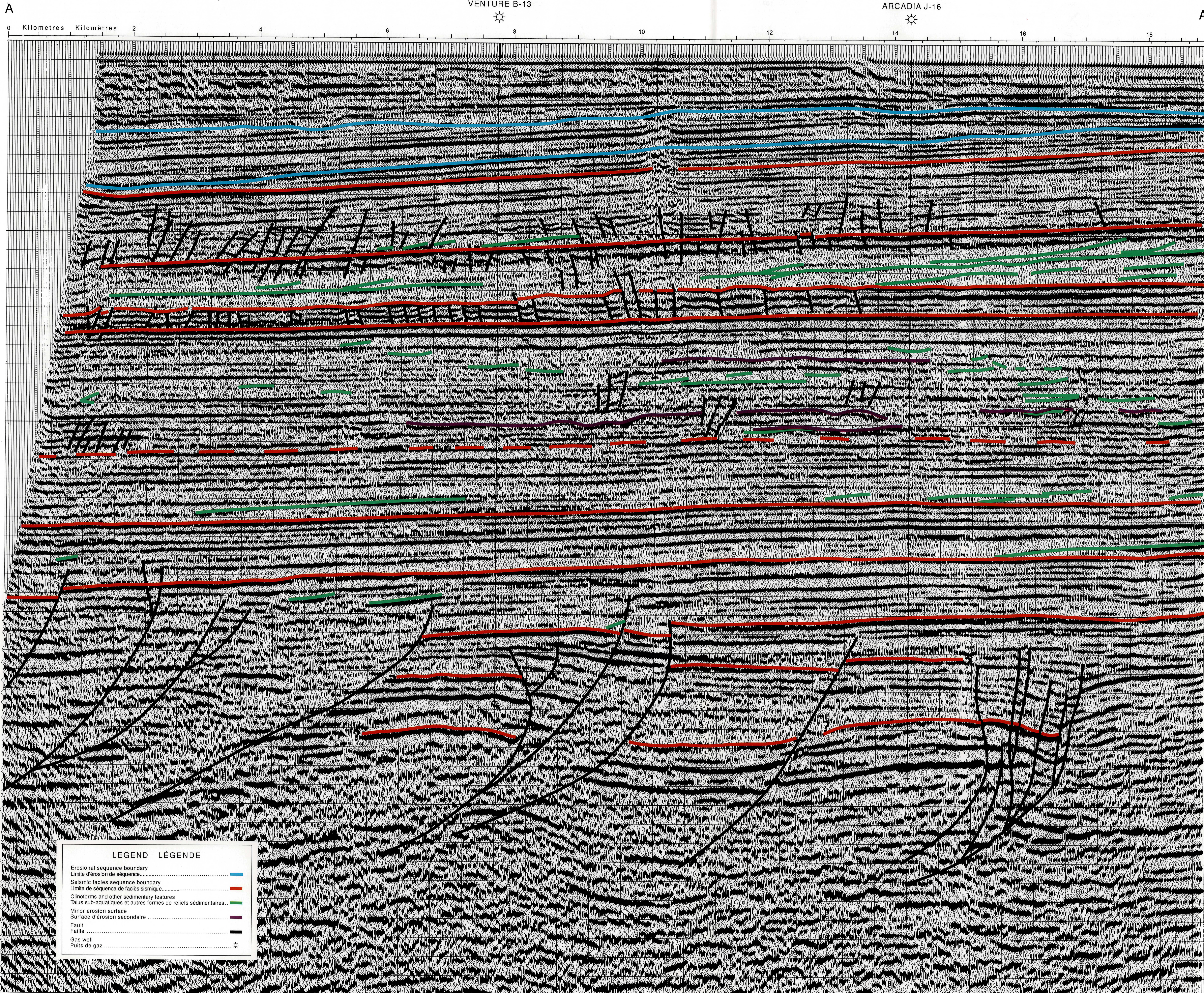
SCOTIAN SHELF SEISMIC EXPRESSION 6 PLATE-FORME NÉO-ÉCOSSAISE SIGNATURE SISMIQUE DETAILED SEISMIC LINE, VENTURE AREA PROFIL SISMIQUE DÉTAILLÉ, RÉGION DE VENTURE
