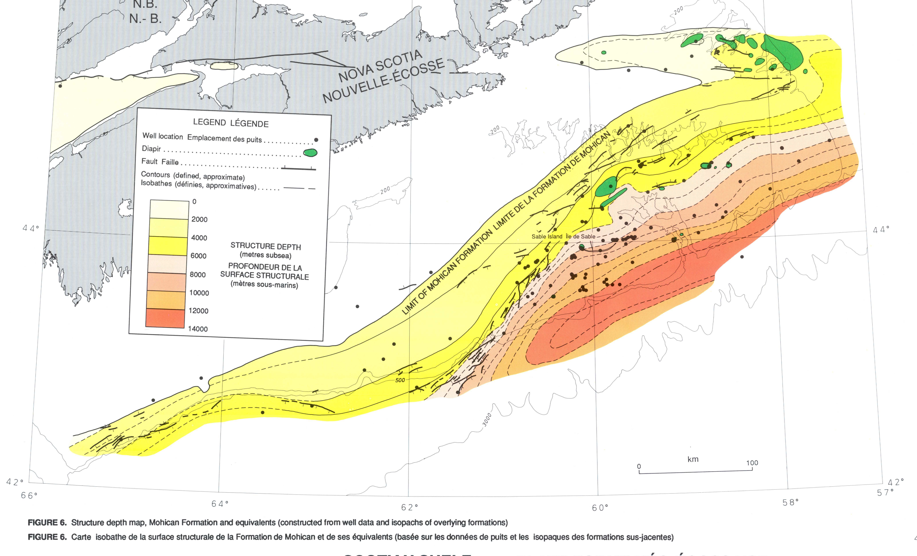
FIGURE 6. Structure depth map, Mohican Formation and equivalents (constructed from well data and isopachs of overlying formations) FIGURE 6. Carte isobathe de la surface structurale de la Formation de Mohican et de ses équivalents (basée sur les données de puits et les isopaches des formations sus-jacentes)
