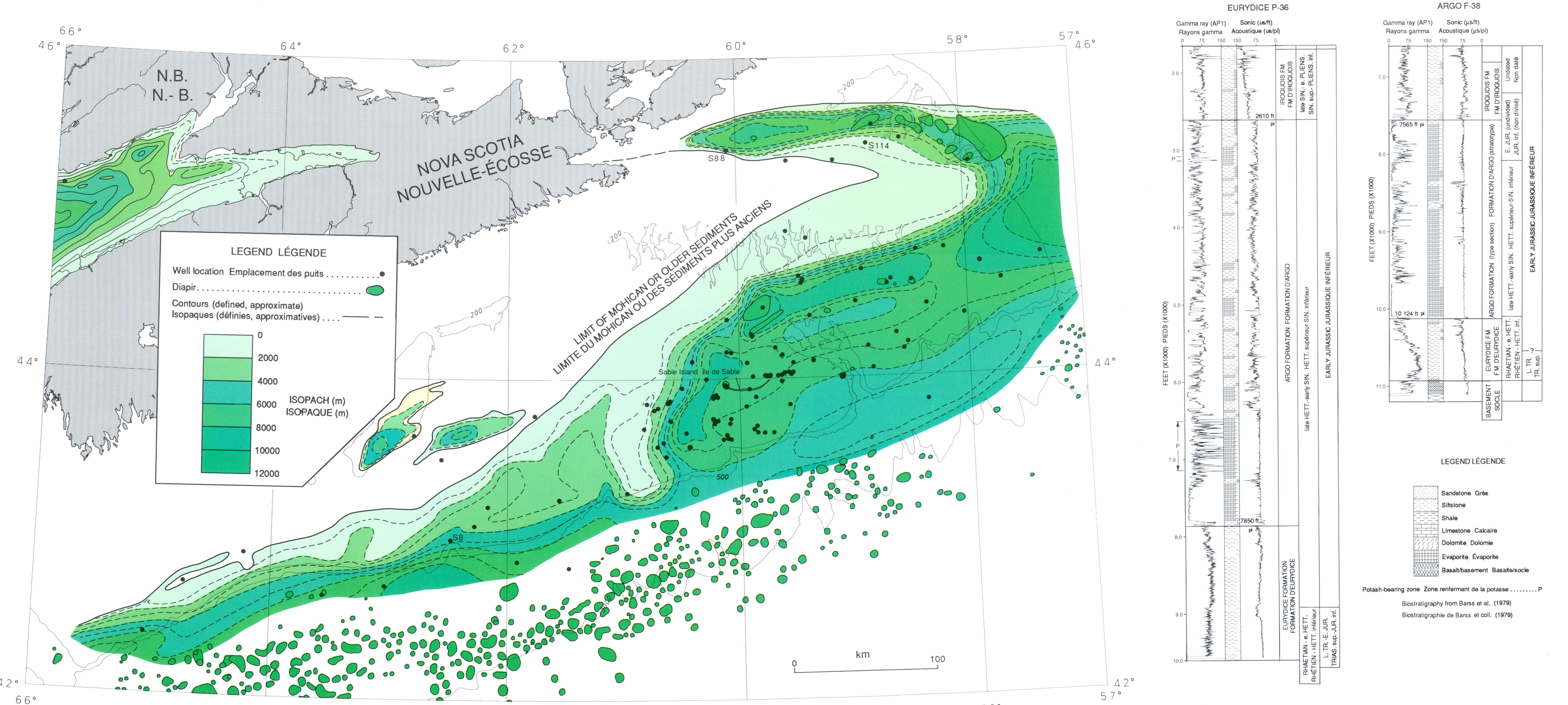
FIGURE 7. Isopach map, top of Mohican Formation to basement (includes Mohican, Iroquois, Argo and Eurydice formations and equivalents) FIGURE 7. Carte isopache, du sommet de la Formation de Mohican jusqu'au socle (ce qui comprend les formations de Mohican, d'Iroquois, d'Argo et d'Eurydice de même que leurs équivalents)
