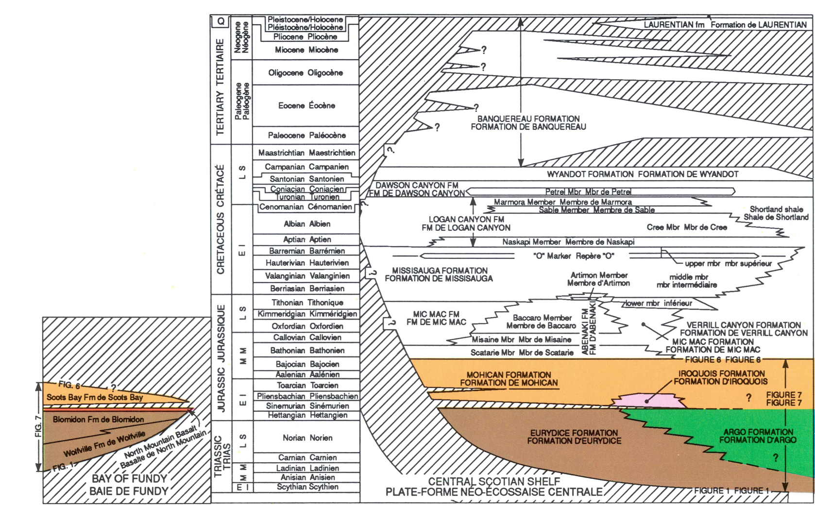
FIGURE 3. Stratigraphie généralisée de la plate-forme Néo-Écossaise centrale montrant le socle pré-mésozoïque, la formation de Mohican ainsi que les formations qui lui sont plus anciennes et leurs équivalents (d'après Wade et MacLean, 1990); la stratigraphie généralisée de la baie de Fundy est également présentée.
