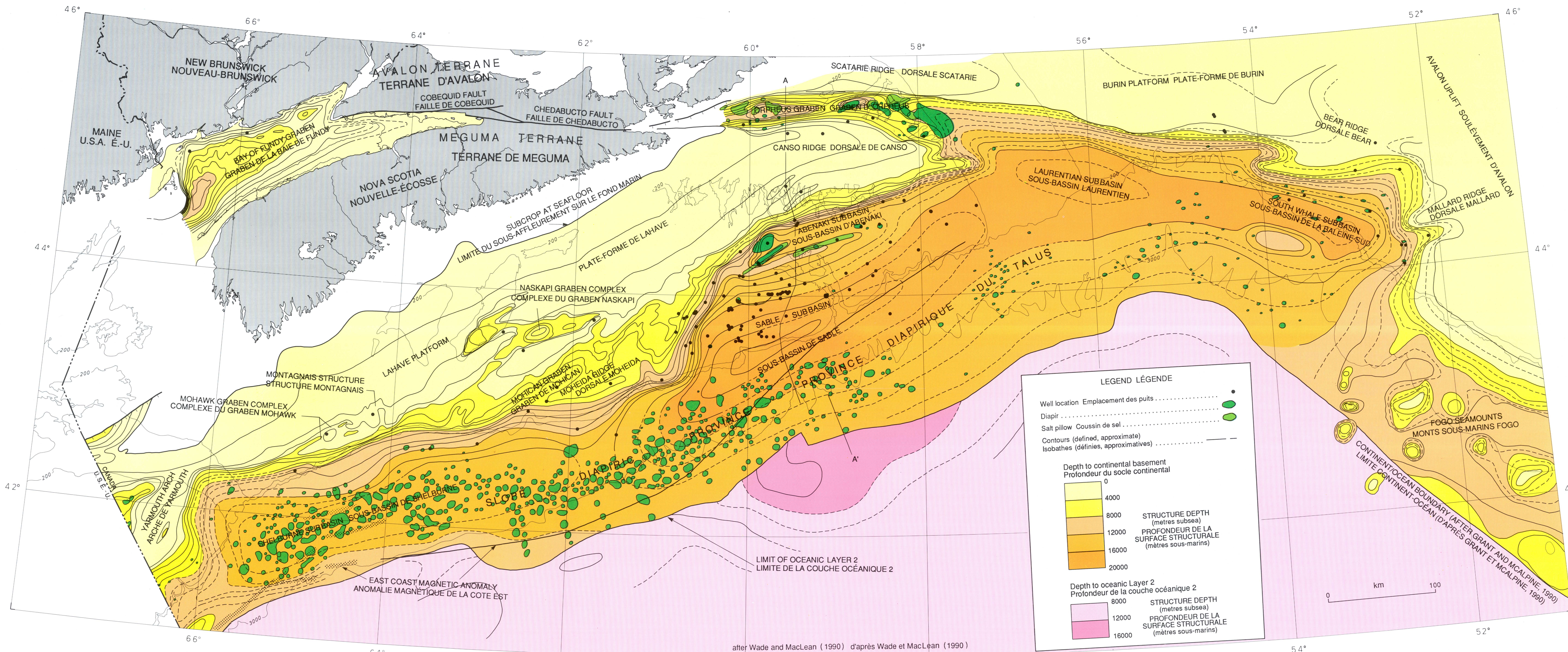
FIGURE 1. Structure depth map, pre-Mesozoic basement FIGURE 1. Carte isobathe de la surface structurale du socle pré-mésozoïque
