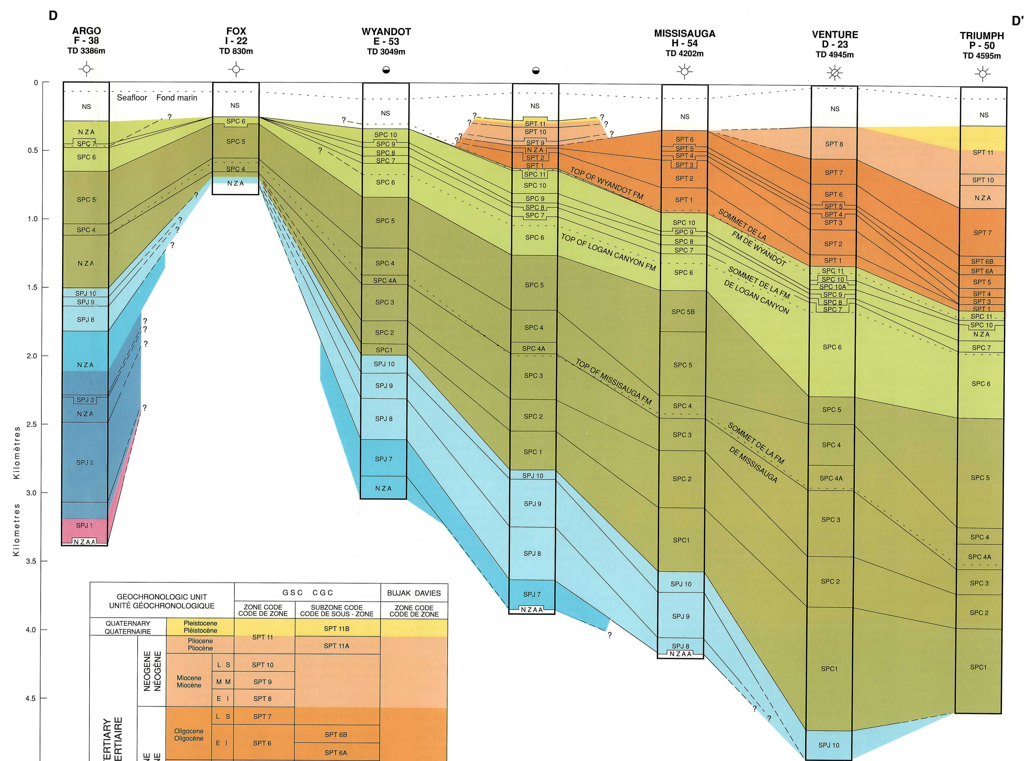
FIGURE 2. Palynostratigraphic cross-section D - D', Argo F-38 to Triumph P-50 FIGURE 2. Coupe palynostratigraphique D - D', Argo F-38 à Triumph P-50
