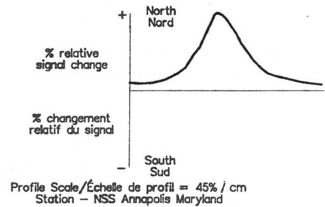
Total field VLF response Réponse VLF du champ total
