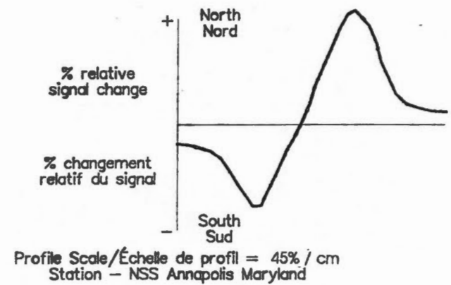
Quadrature VLF response Réponse Quadrature VLF
