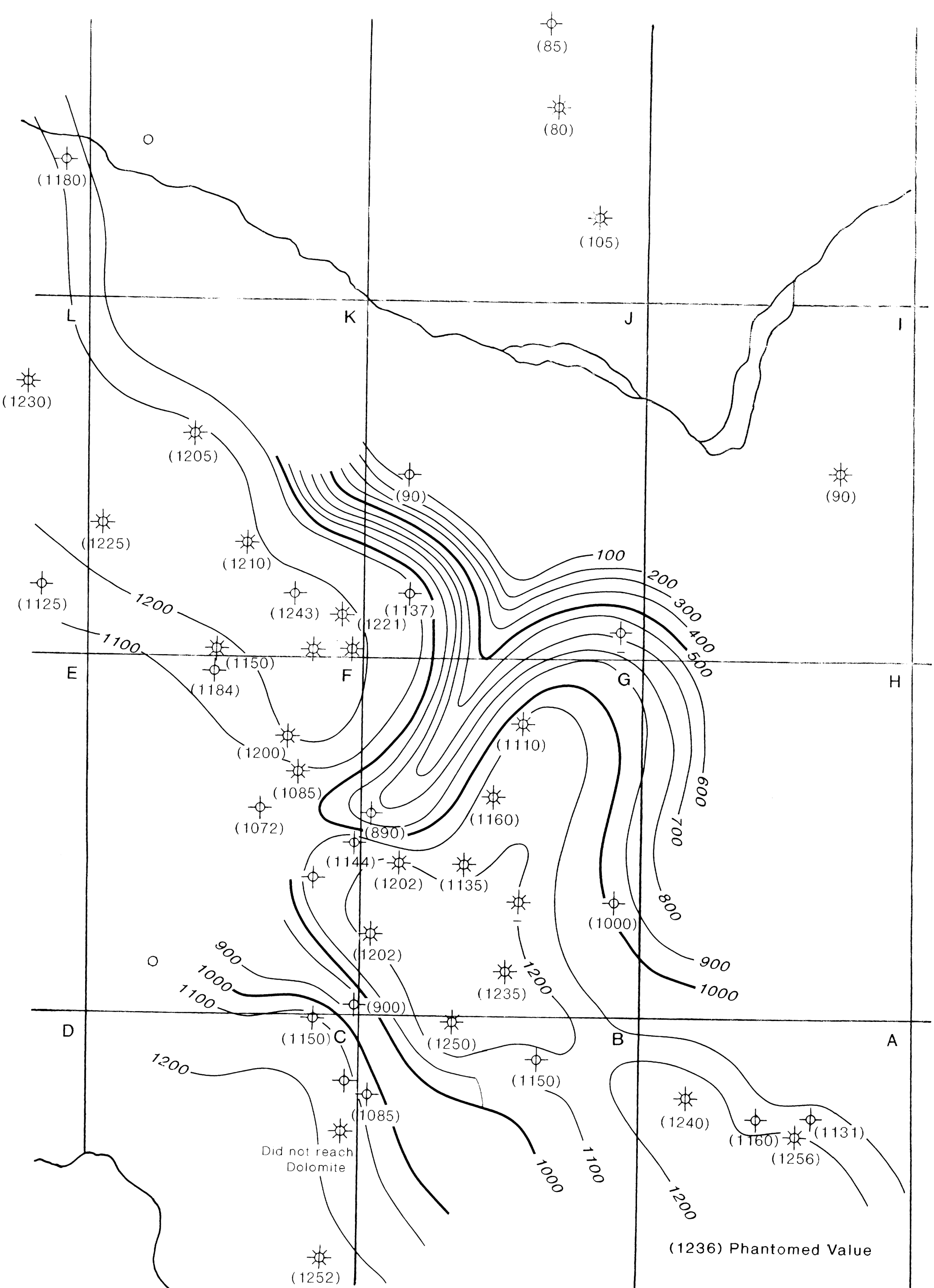
Top Presqu'ile Dolomite to Chinchaga (Feet) CI - 100 Feet
