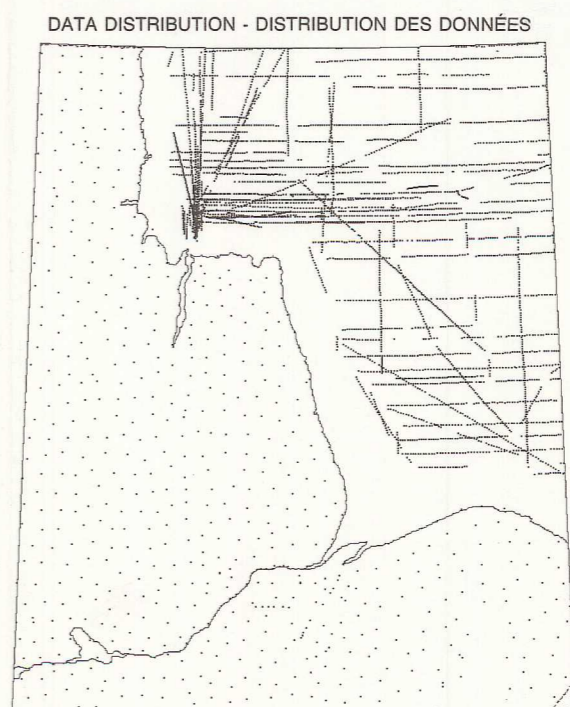
NATIONAL EARTH SCIENCE SERIES SÉRIE NATIONALE DE LA SCIENCE DE LA TERRE MAP - CARTE NO-15-GR (BA) CHURCHILL
