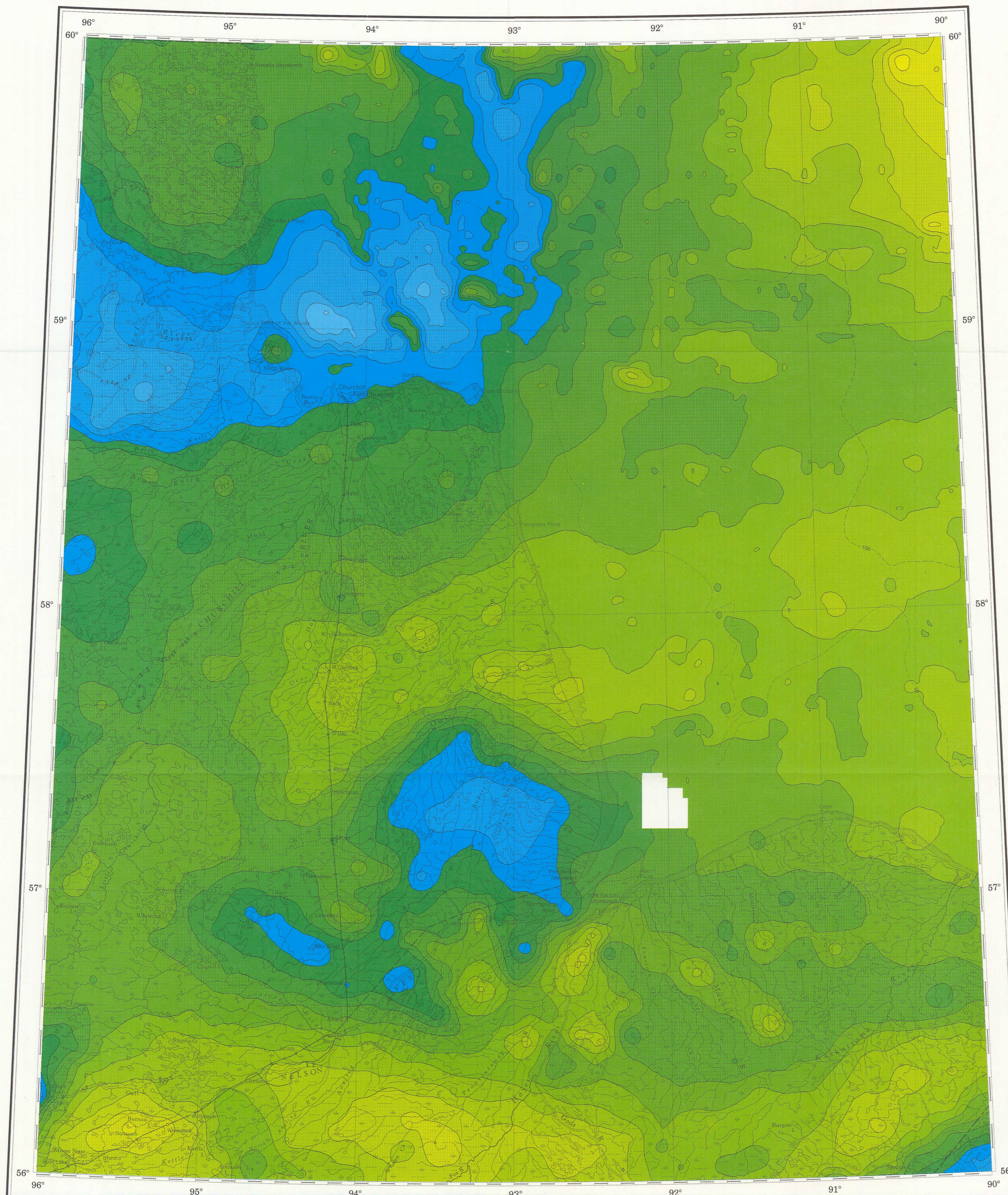
MAP NO-15-GR (BA) CARTE GRAVITY - BOUGUER ANOMALIES - GRAVITÉ - ANOMALIES DE BOUGUER
