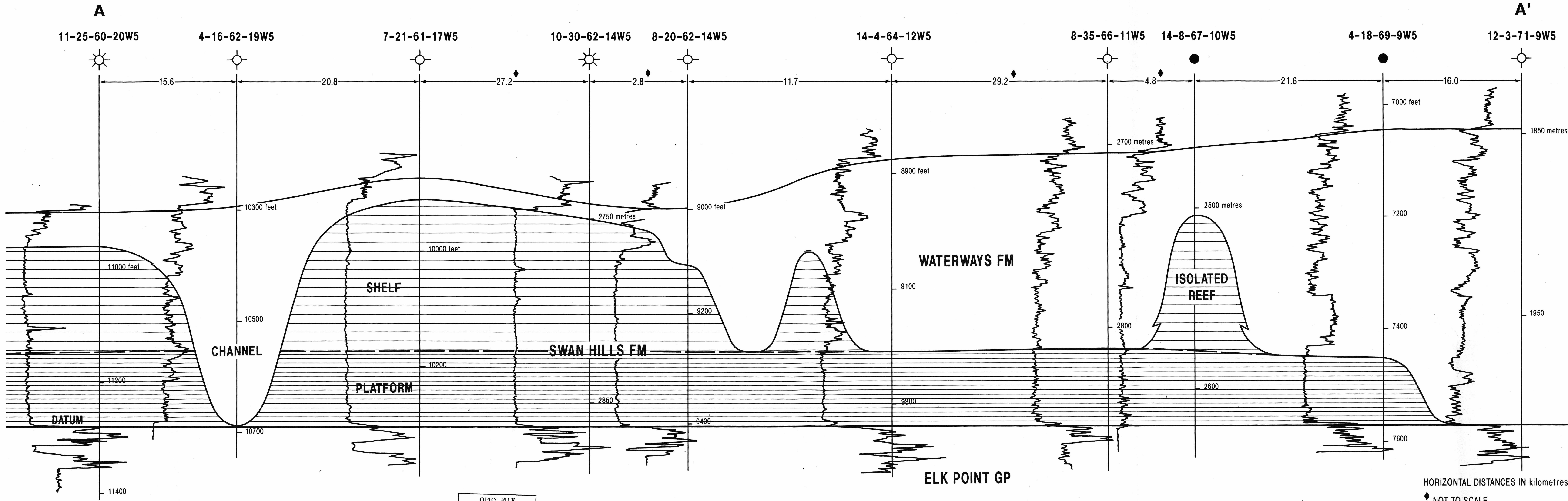
FIGURE 2 CROSS SECTION A - A' SWAN HILLS FORMATION Figure 2. Coupe stratigraphique A-A' de la Formation de Swan Hills
