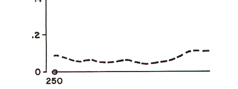
QUADRATURE PROFILE PROFIL DE QUADRATURE Solid line is total field VLF Scale is 1 cm = 20% Le trait continu représente le champ total TBF L'échelle est de 1 cm = 20%
