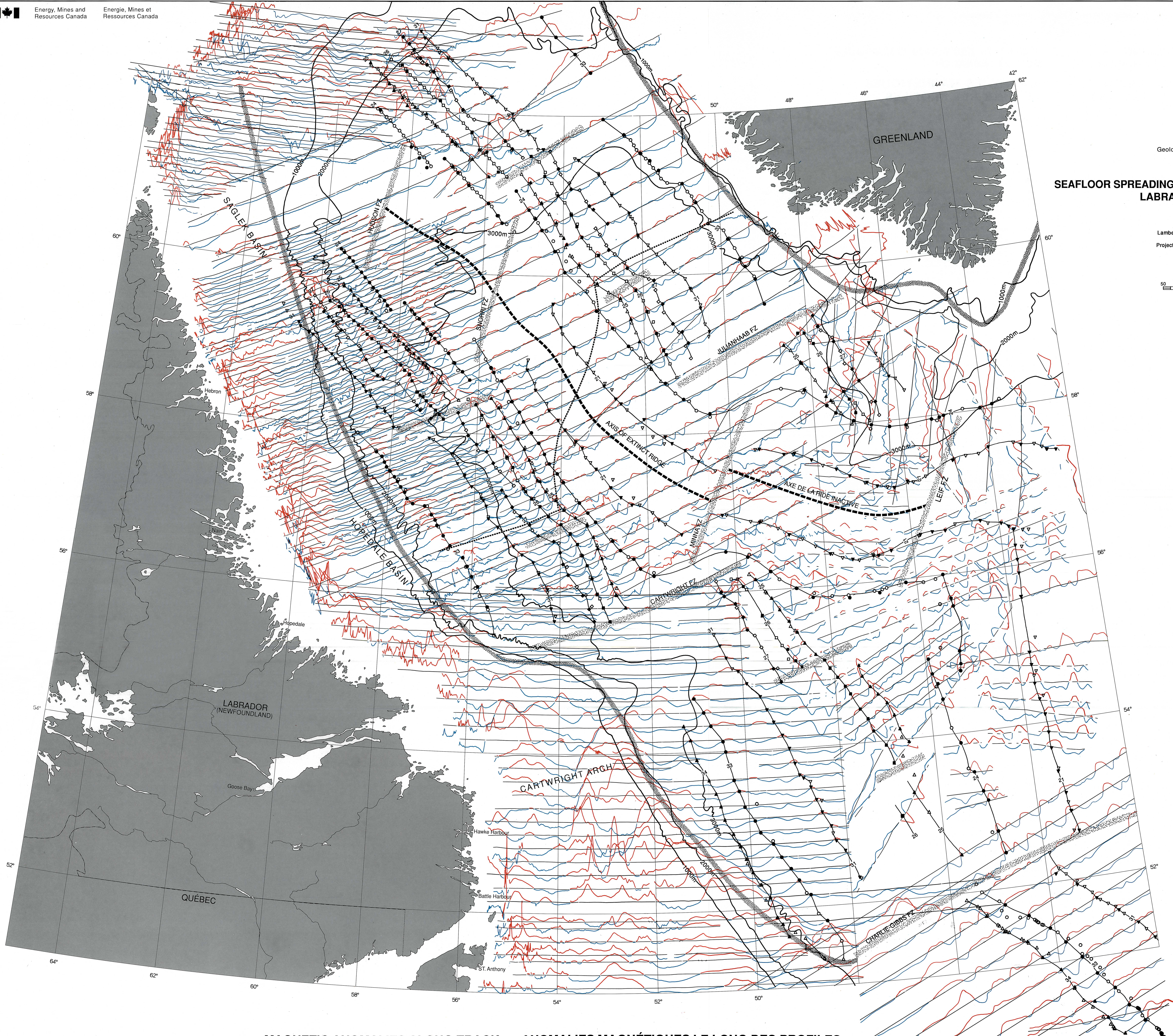
MAGNETIC ANOMALIES ALONG TRACK | ANOMALIES MAGNÉTIQUES LE LONG DES PROFILES
