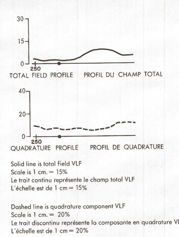
TOTEM VLF EM PROFILES FOR LINE STATION PROFILS DE TOTEM EM VLF POUR LA STATION EN LIGNE
