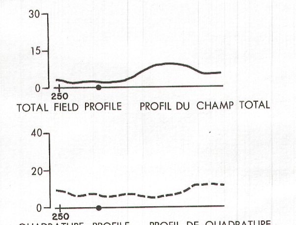
TOTEM VLF EN PROFILS POUR LINE STATION PROFILS DE TOTEM EN VLF POUR LA STATION EN UJONE
