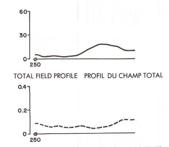
Solid line is total field VLF Scale is 1 cm = 30% Le trait continu représente le champ total VLF L'échelle est de 1 cm = 30% Dashed line is quadrature component VLF Scale is 1 cm = 0.2%/m Le trait discontinu représente la composante en quadrature VLF L'échelle est de 1 cm = 0.2%/m
