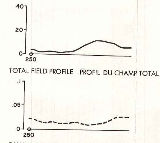
TOTAL FIELD PROFILE PROFIL DU CHAMP TOTAL Solid line is total field VLF Scale is 1 cm = 20% Le trait continu représente le champ total VLF L'échelle est de 1 cm = 20% QUADRATURE PROFILE PROFIL DE QUADRATURE Dashed line is quadrature component VLF Scale is 1 cm = .05%/m Le trait discontinu représente la composante en quadrature VLF L'échelle est de 1 cm = .05%/m
