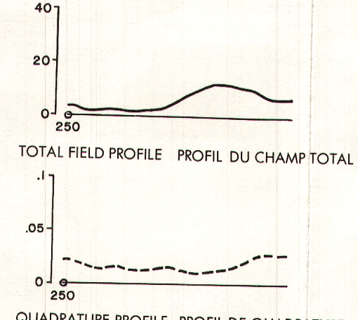
TOTAL FIELD PROFILE PROFIL DU CHAMP TOTAL QUADRATURE PROFILE PROFIL DE QUADRATURE Solid line is total field VLF Scale is 1 cm = 20% Le trait continu représente le champ total VLF L'échelle est de 1 cm = 20% Dashed line is quadrature component VLF Scale is 1 cm = .05% / m Le trait discontinu représente la composante en quadrature VLF L'échelle est de 1 cm = .05% / m
