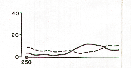
TOTEM VLF EM TOTAL FIELD PROFILES PROFILS DU CHAMP TOTAL TOTEM EM VLF
