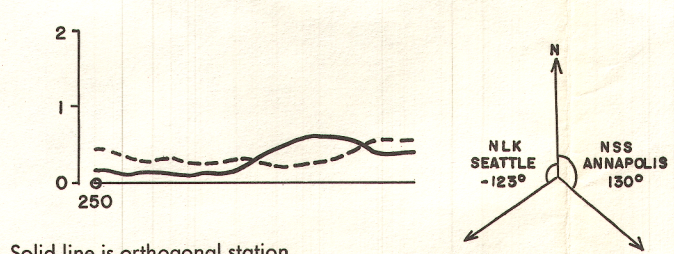
TOTEM VLF EM QUADRATURE PROFILES PROFILS DE QUADRATURE TOTEM EM VLF
