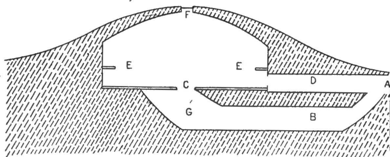
Figure 1. Coupe perpendiculaire du kázgi de St-Michel.
