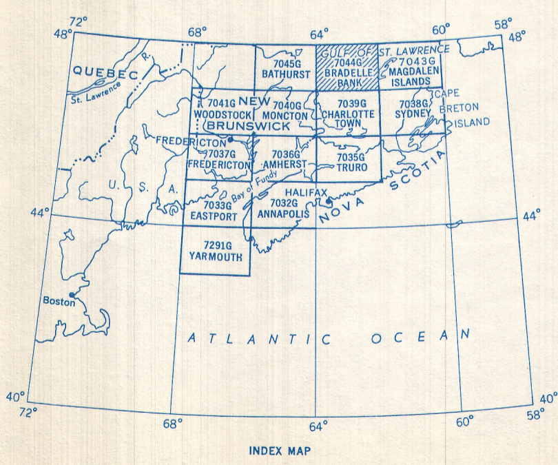
INDEX MAP
