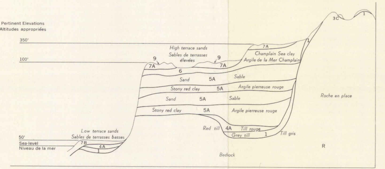
DIAGRAMMATIC RELATIONSHIP OF STRATIGRAPHY TO TOPOGRAPHY SCHEMA MONTRANT LE RAPPORT ENTRE LA STRATIGRAPHIE ET LA TOPOGRAPHIE
